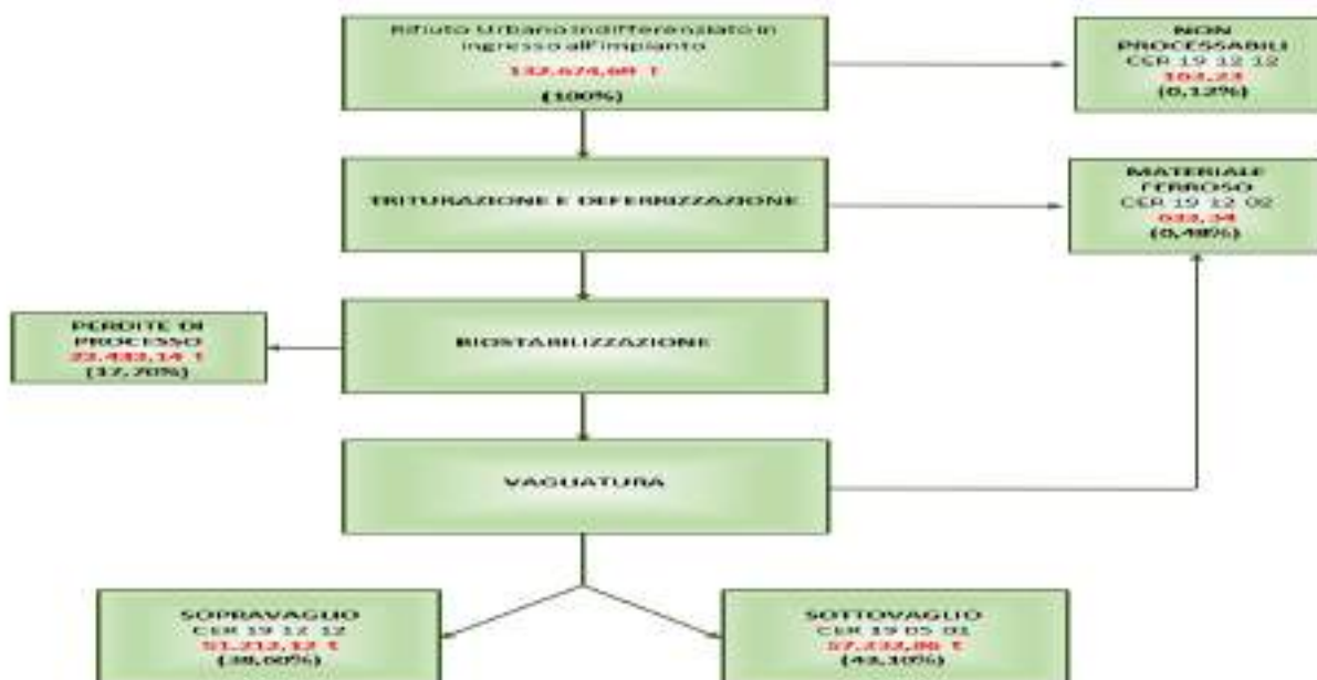
Figura 4: Bilancio di massa dell'impianto TMB di Foggia, relativo all'anno 2023.
