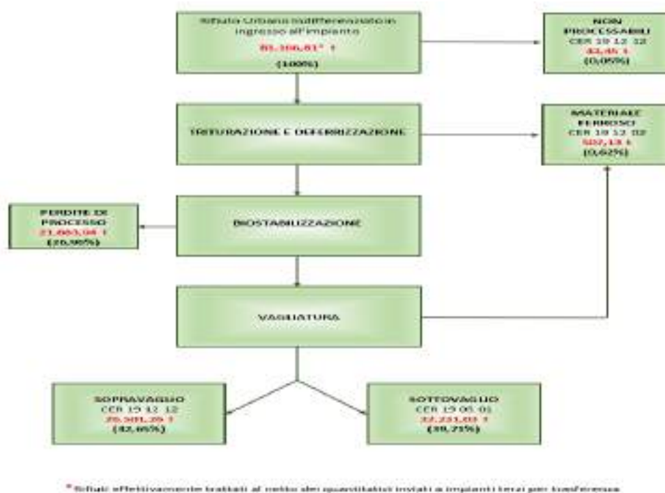
Figura 2: Bilancio di massa dell'impianto TMB di Bari, relativo all'anno 2023.
